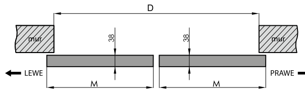
system podwójny
